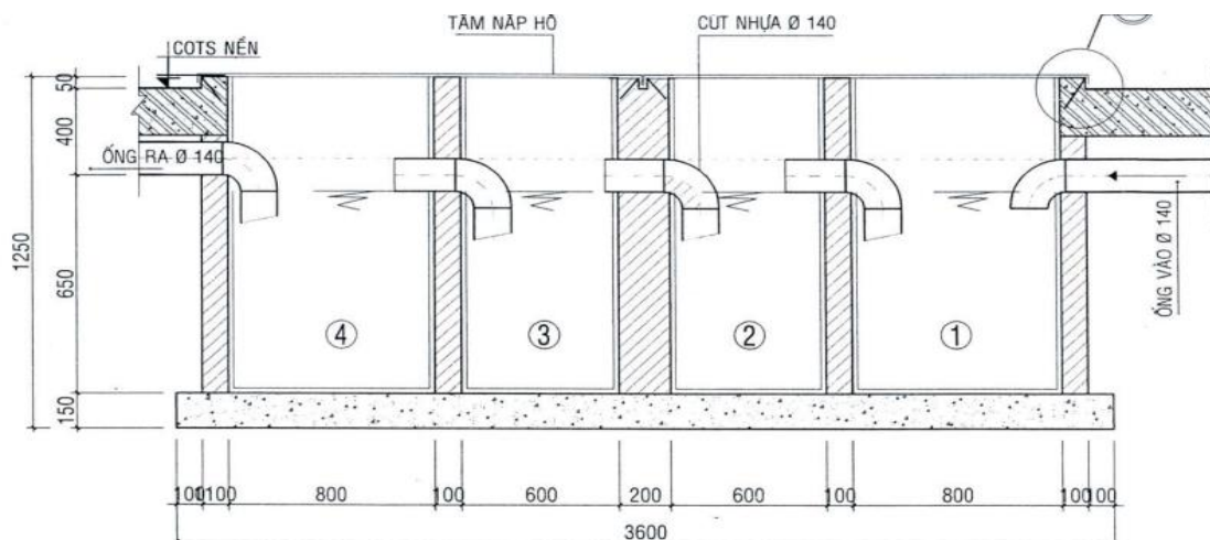
Hình 3.1. Sơ đồ xử lý nước mưa (nước thải) nhiễm dầu
