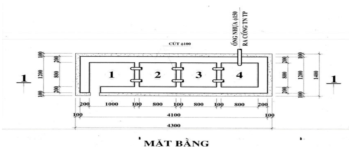
Hình 3.2. Mô hình bể tách dầu 4 ngăn
