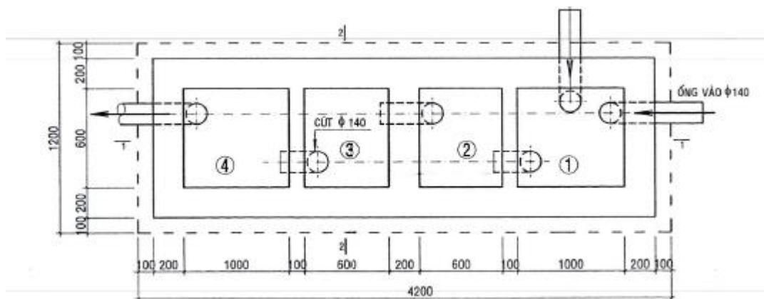
Hình 3.2. Mô hình bể tách dầu 4 ngăn
